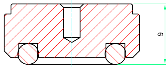
A-A (3:1)
