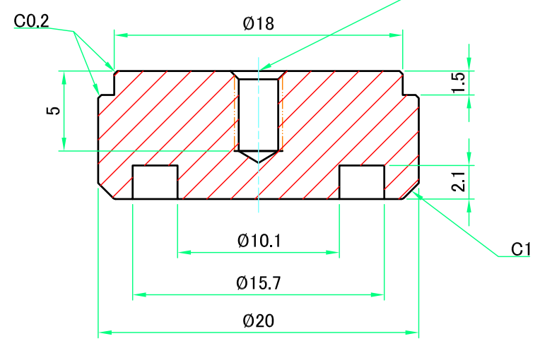
B-B (3:1)
