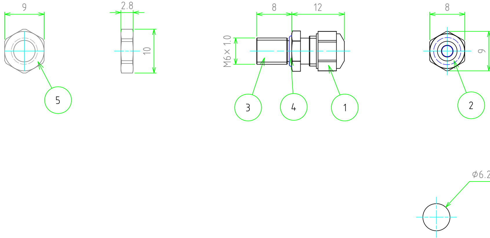
取付穴寸法 / Mounting hole dimensions
