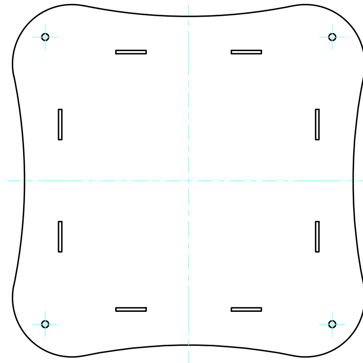
下カバー裏面 / Bottom cover Backside
