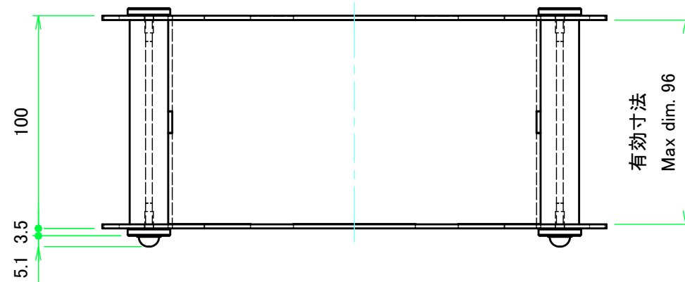
Wパネル1 / W Panel 1
