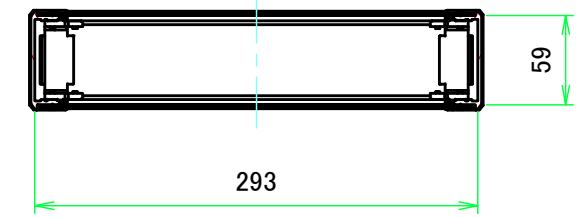
C-C ( 1:5 )
