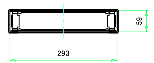
C-C ( 1:6 )
