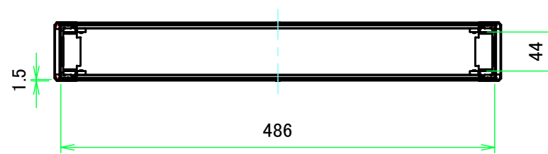
A-A ( 1:6 )
