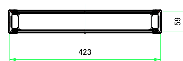
C-C ( 1:6.5 )
