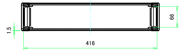
A-A (1:5)
