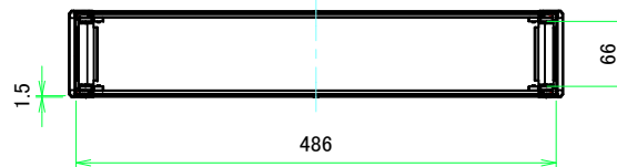
A-A (1:6)
