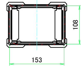
C-C ( 1 : 5.5 )
