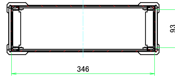
A-A ( 1 : 5.5 )
