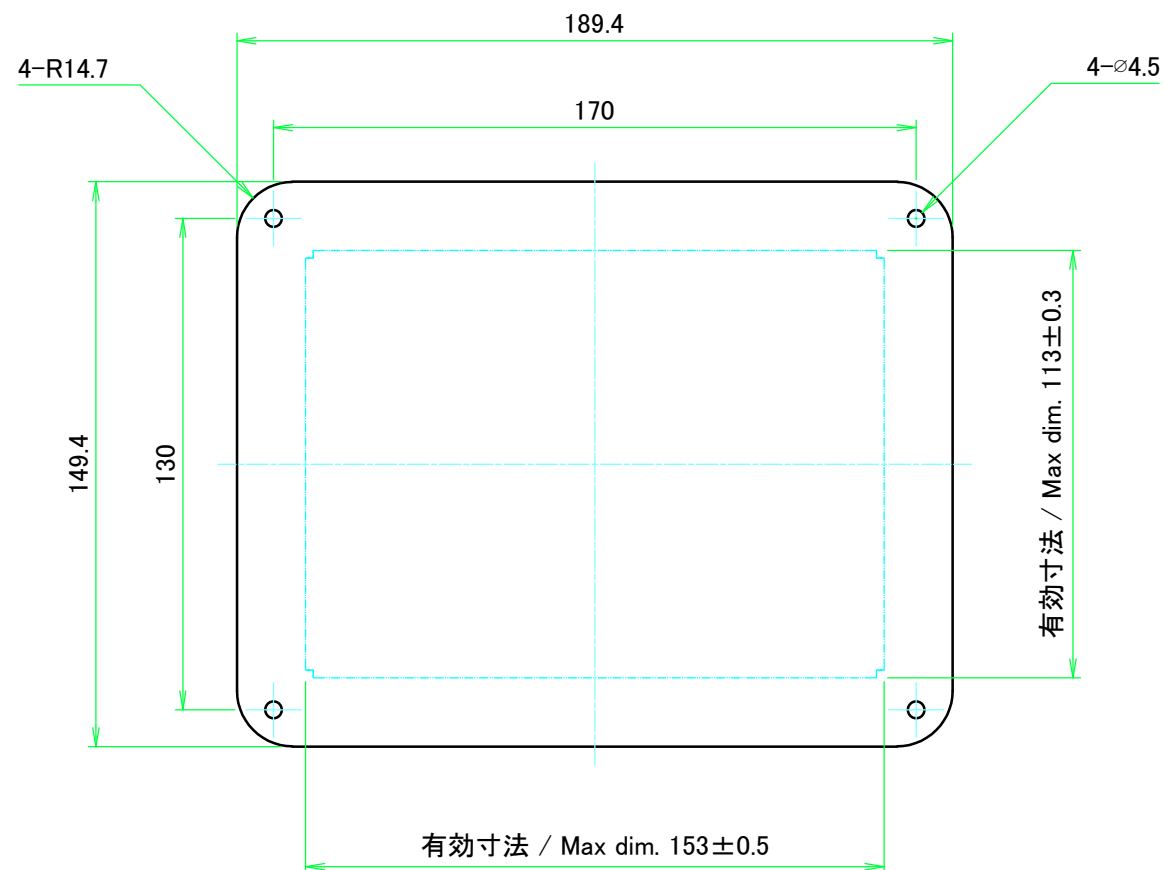
保護シート側 Surface protective film side
