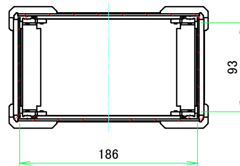
A-A (1:4)
