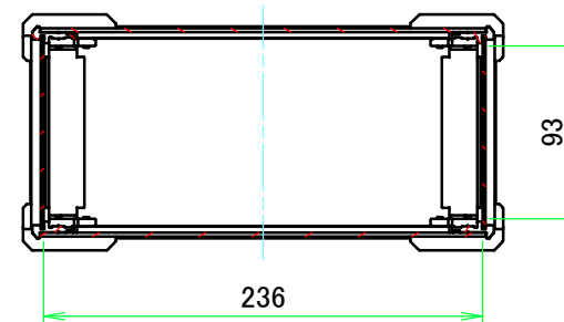
A-A ( 1 : 4.5 )
