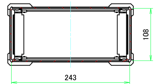
C-C ( 1 : 4.5 )
