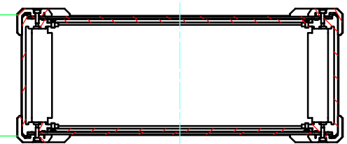
D-D (1:5)
