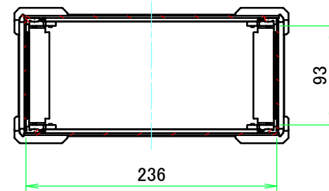
A-A (1:5)
