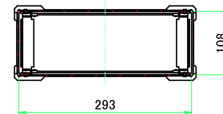
C-C ( 1 : 6.5 )
