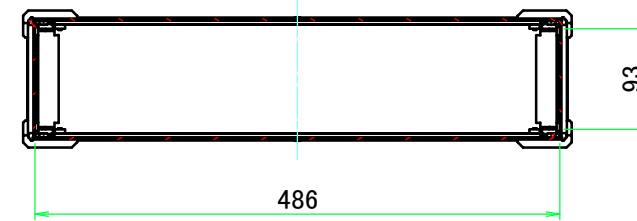
A-A (1:7)
