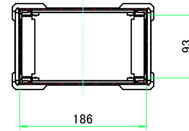
A-A ( 1 : 5.5 )
