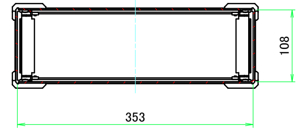
C-C ( 1 : 5.5 )
