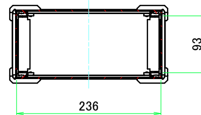
A-A (1:6)
