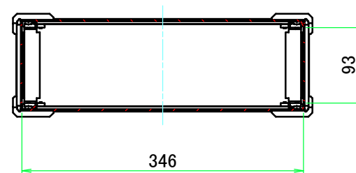
A-A ( 1 : 6.5 )
