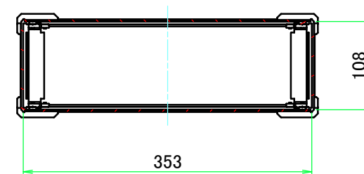
C-C ( 1 : 6.5 )
