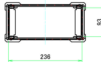
A-A (1:6)
