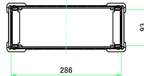
A-A (1:6)
