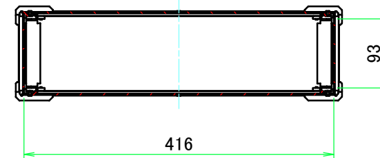
A-A (1:7)
