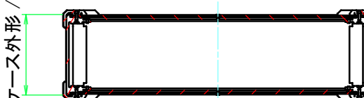
D-D (1:7.5)
