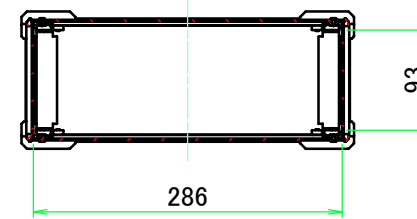
A-A (1:7)
