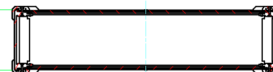
D-D (1:7)
