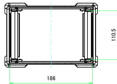
A-A ( 1:3.5 )
