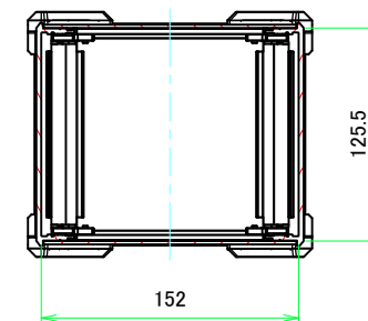
C-C ( 1:3.5 )
