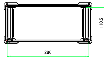
A-A ( 1:4.5 )
