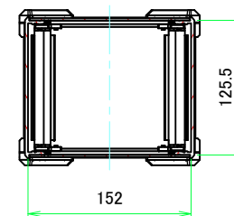
C-C ( 1:4.5 )
