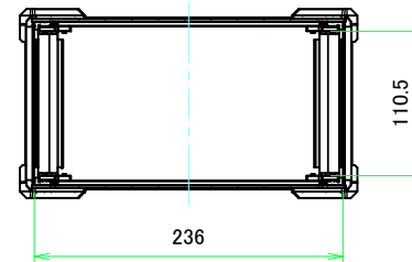
A-A ( 1:4.5 )
