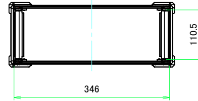
A-A ( 1:6 )
