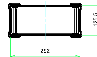
C-C ( 1:7 )
