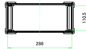
A-A (1:6)
