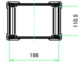
A-A (1:6)
