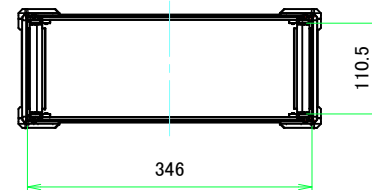
A-A (1:6.5)
