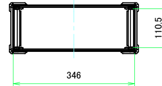
A-A (1:7.5)
