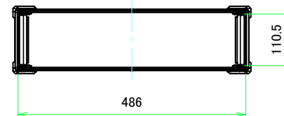
A-A (1:8)
