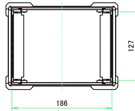
A-A (1:4)
