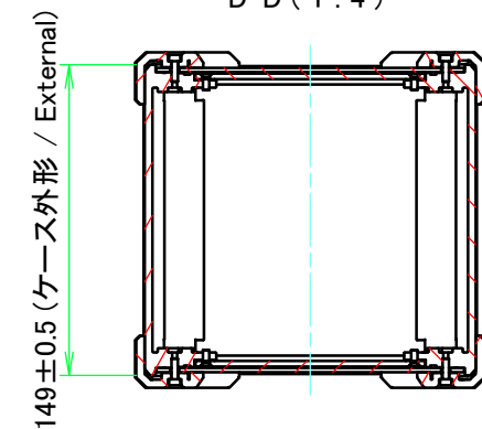
D-D (1:4)
