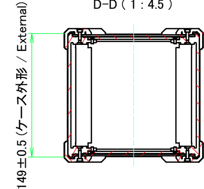
D-D (1:4.5)
