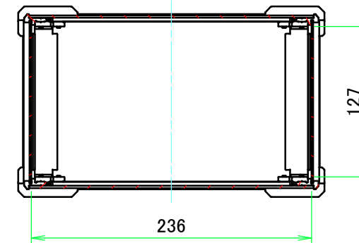
A-A (1:4.5)
