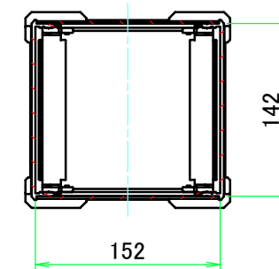
C-C ( 1 : 5.5 )
