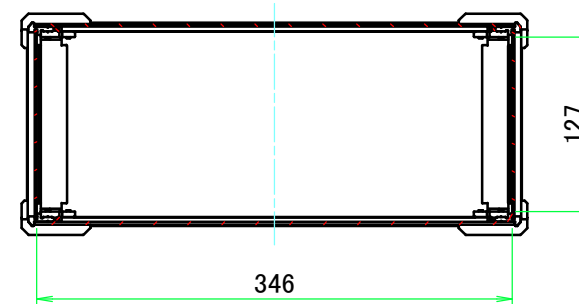
A-A ( 1 : 5.5 )
