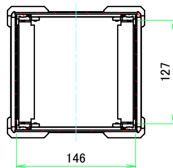
A-A ( 1 : 4.5 )
