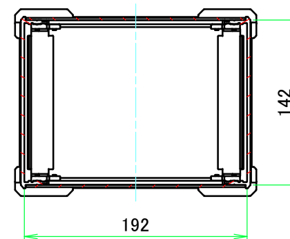
C-C ( 1 : 4.5 )
