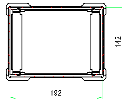
C-C ( 1 : 4.5 )
