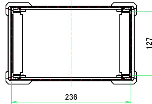
A-A ( 1 : 4.5 )
