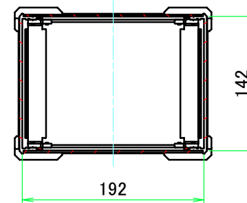
C-C ( 1 : 5.5 )
