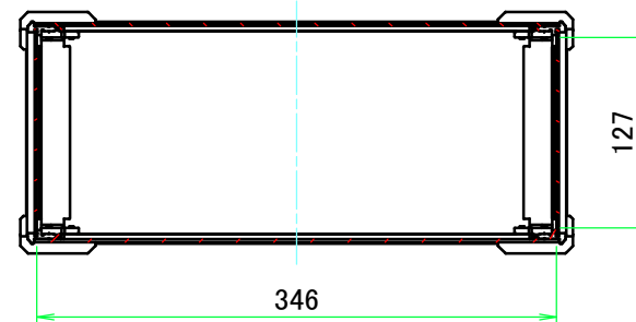
A-A ( 1 : 5.5 )
