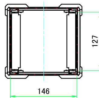
A-A (1:5)
