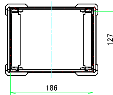
A-A (1:5)
