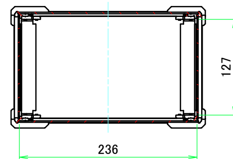
A-A (1:5)
