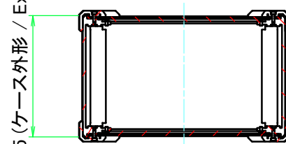
D-D ( 1 : 6.5 )
