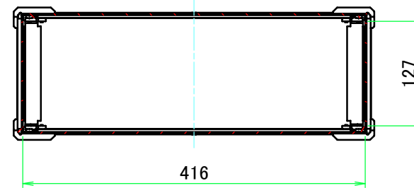
A-A ( 1 : 6.5 )
