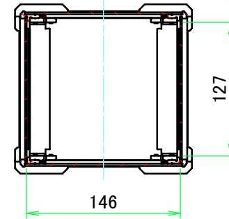
A-A (1:5)
