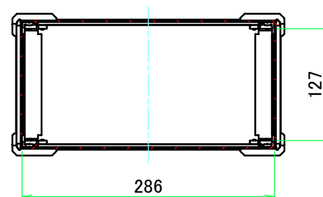
A-A (1:6)
