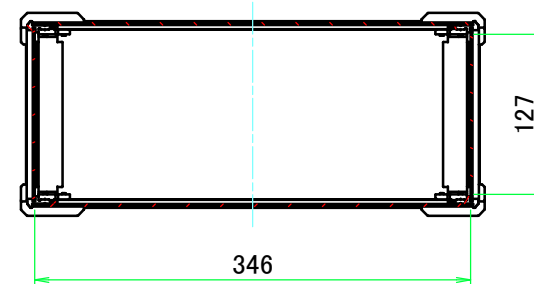
A-A (1:6)
