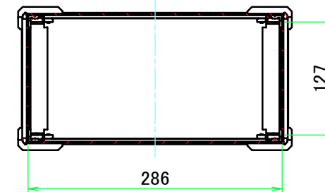
A-A (1:6)
