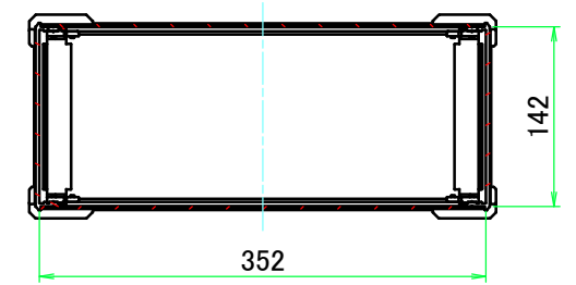
C-C ( 1 : 6.5 )
