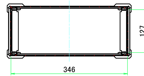
A-A ( 1 : 6.5 )
